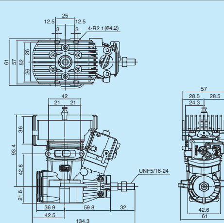
寸法図 (単位 mm) Dimensions (mm)
