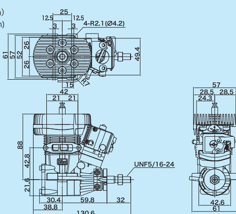
寸法図 (単位 mm) Dimensions (mm)
