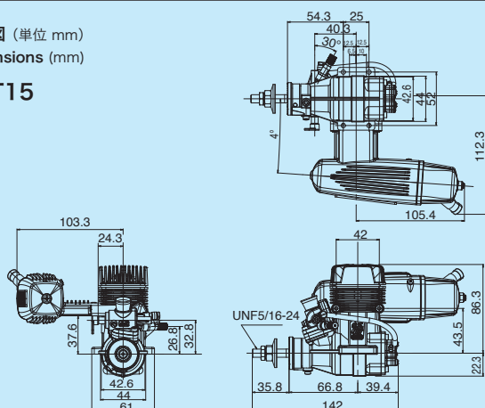
寸法図 (単位 mm) Dimensions (mm)
