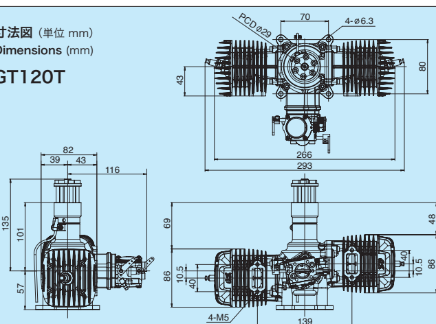
寸法図 (単位 mm) Dimensions (mm)
