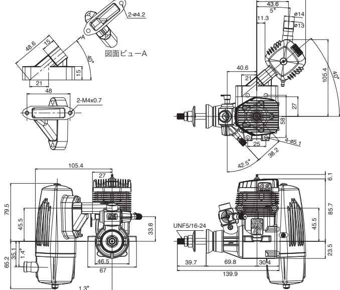
90°アダプター装着図
