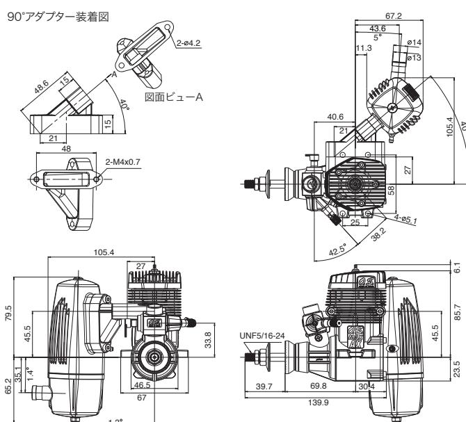
90°アダプター装着図
