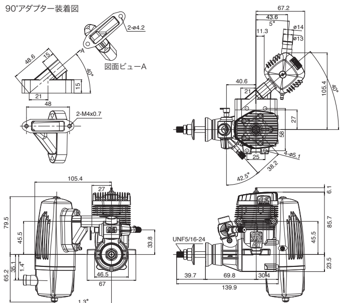
90°アダプター装着図
