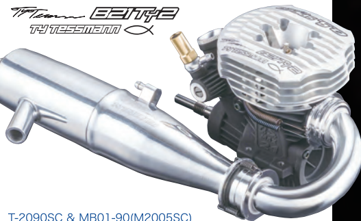
T-2090SC & MB01-90(M2005SC)
