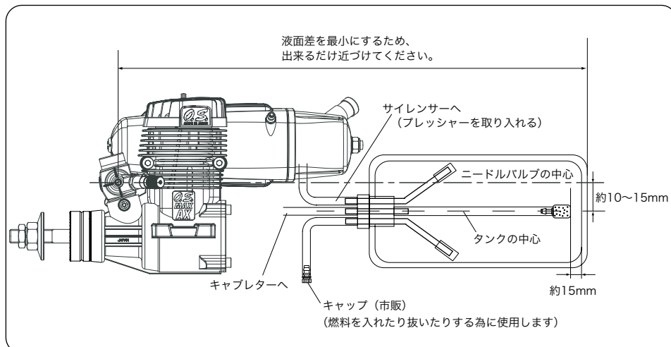
燃料タンクの配管及び位置 (参考図)
