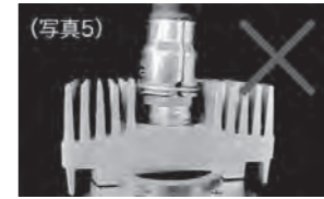
不完全な取り付け状態1 (写真5) (ノイズ発生、誤動作の主な原因)
