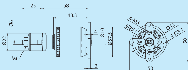
寸法図 (単位:mm) OMA-3820-1200 Dimensions (mm)
